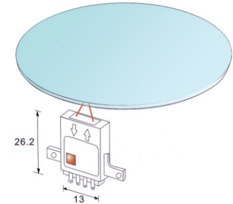
微型光电传感器 Micro photoelectric sensor
