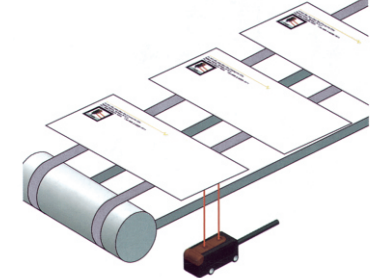
微型方形光电传感器 Micro-sized square photoelectric sensor
