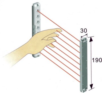
安全光幕传感器 Safety Light Curtain
