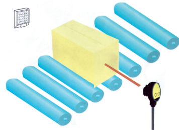
扩散反射式红外线传感器 Diffuse reflective infrared sensors
